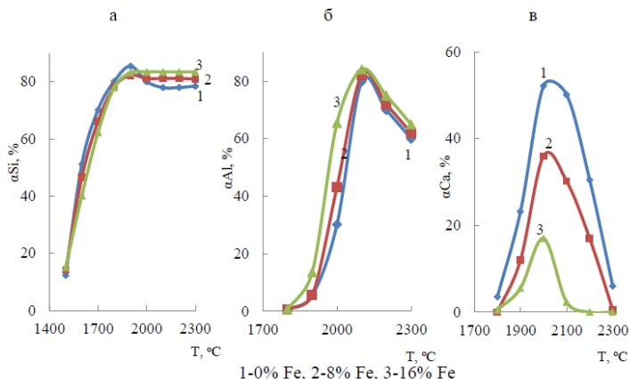
Рисунок 1. Влияние железа на равновесную степень распределения Si (а), Al(б) в сплав и Ca (в) в карбид кальция в системе ОБ-40%C- Fe
