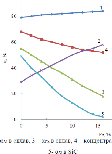
Рисунок 3. Влияние железа на технологические показатели получения ферросплава и карбида кальция при 2000оС из смеси опоки и базальта
